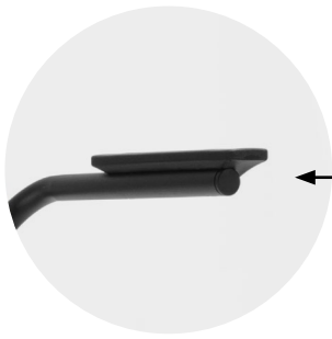
PU armrest
